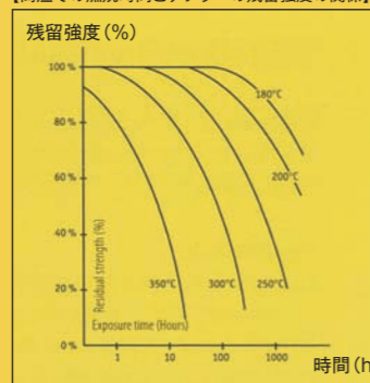
【高温での燃焼時間とケブラーの残留強度の関係】
